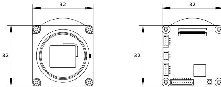
底视图尺寸
