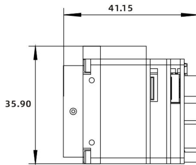
侧视图尺寸
